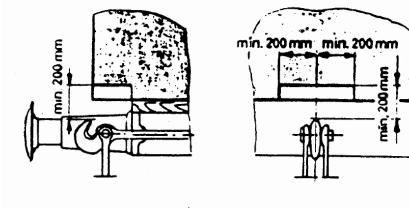
Fig. A7 Freiraum an den Wagenenden über dem Zughaken
